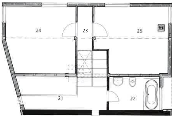
Pôdorys 2, NP 21 – schodisková medzipodesta, knižnica, 22 – kúpeľňa, WC, 23 – chodba, 24 – spálňa, 25 – spálňa
