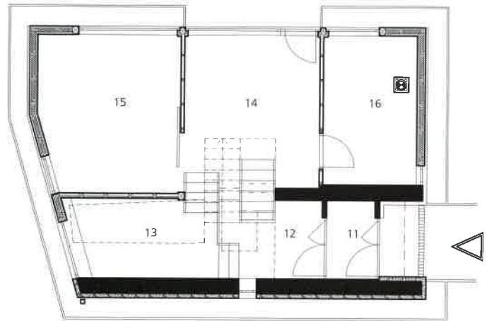
Pôdorys 1, NP 11 – zádverie, 12 – chodba, 13 – knižnica, 14 – obývačka, 15 – kuchyňa, 16 – hosťovská izba
